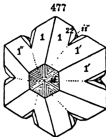
Alexandrite.
